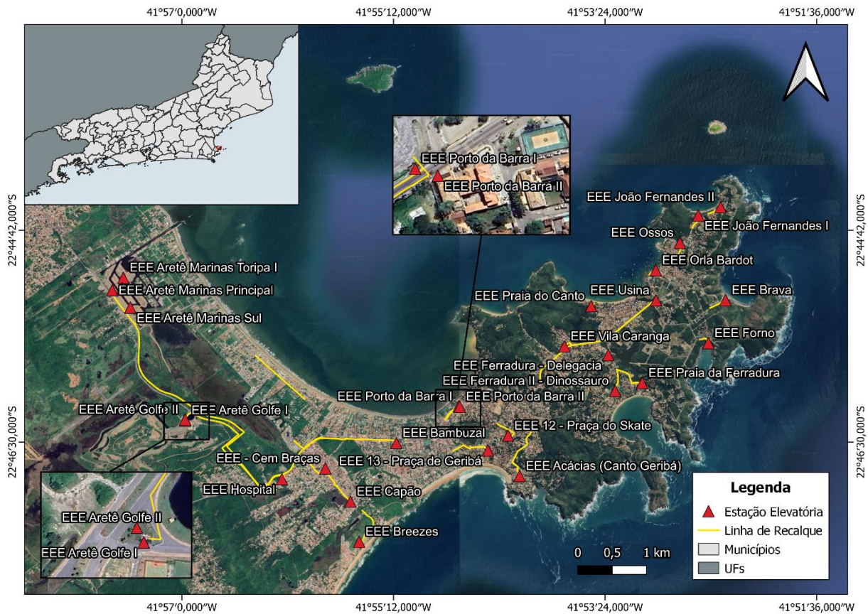
Figura 48 – Estações Elevatórias de Esgoto e Linhas de Recalque – Armação dos Búzios.
