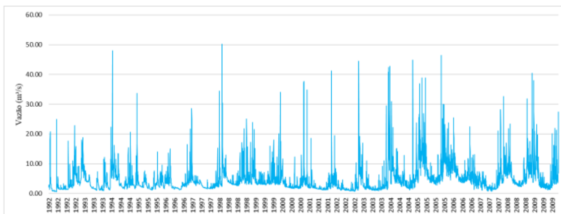
Figura 27 - Hidrograma de vazões simuladas para a sub-bacia Armação dos Búzios.
