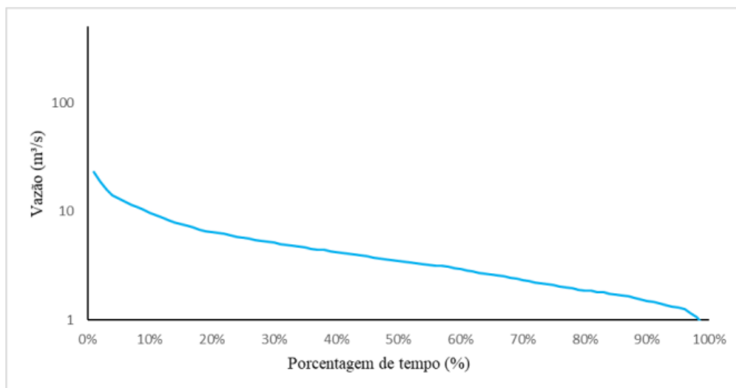
Figura 28 - Curva de permanência.
