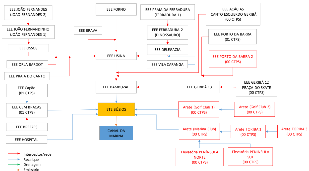
Figura 51 - Fluxograma SES Armação dos Búzios.
