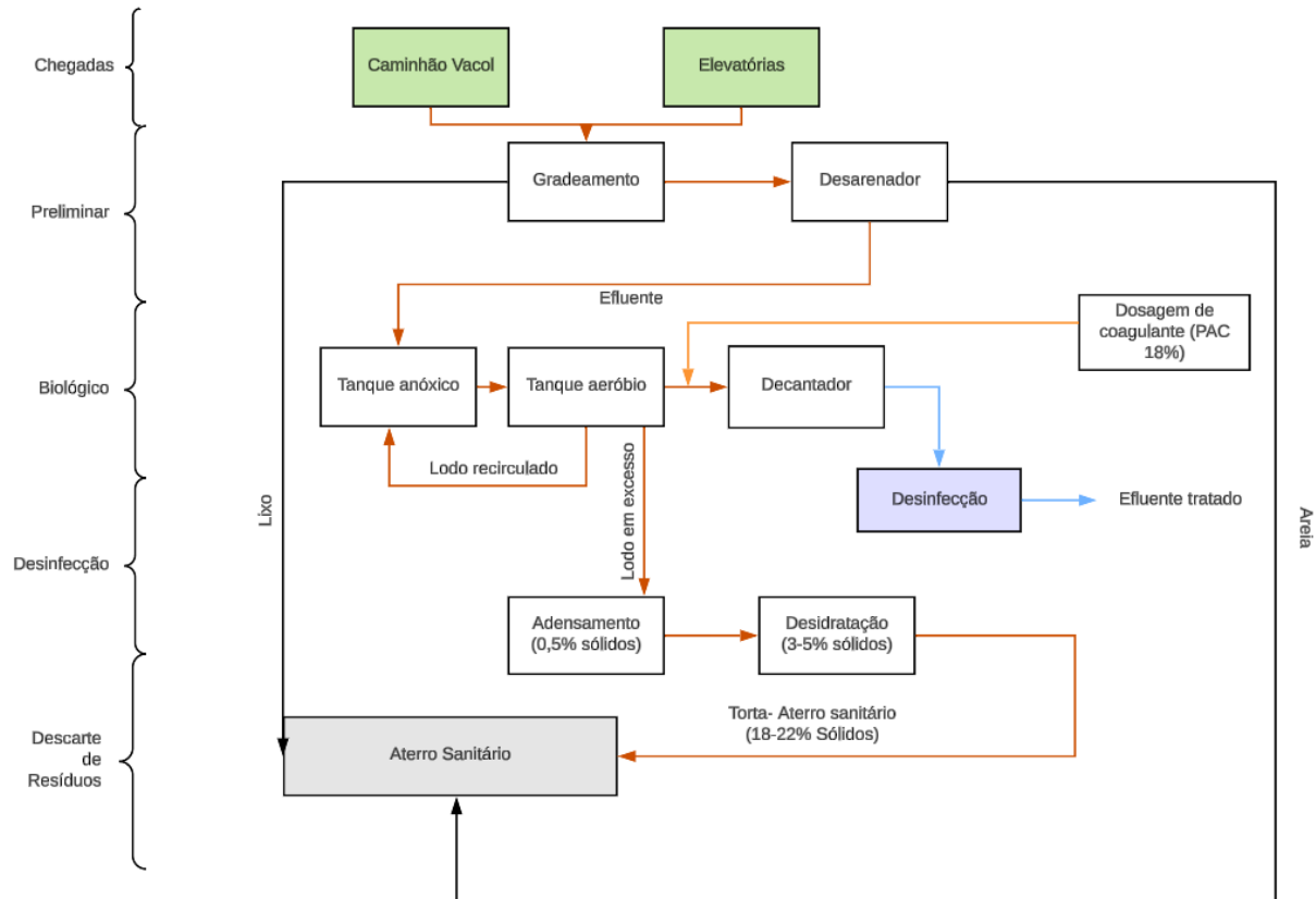
Figura 50 – Fluxograma ETE Búzios.
