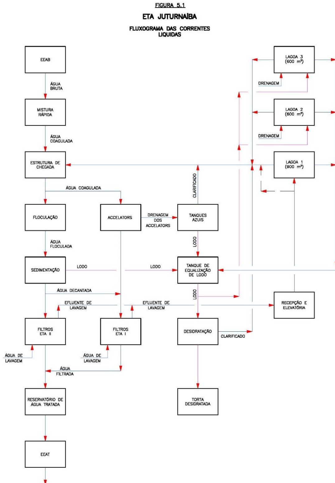
Figura 43 – Fluxograma ETA Juturnaíba.
