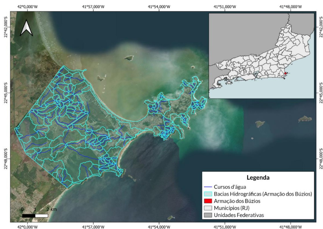
Figura 70 - Bacias Hidrográficas de Armação dos Búzios.
